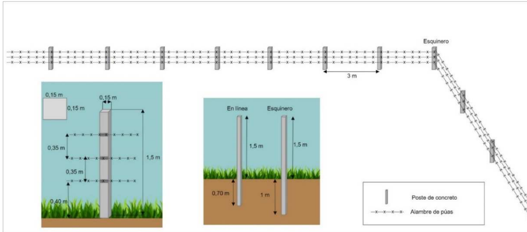
Figura 12-10 Modelo cerramiento
