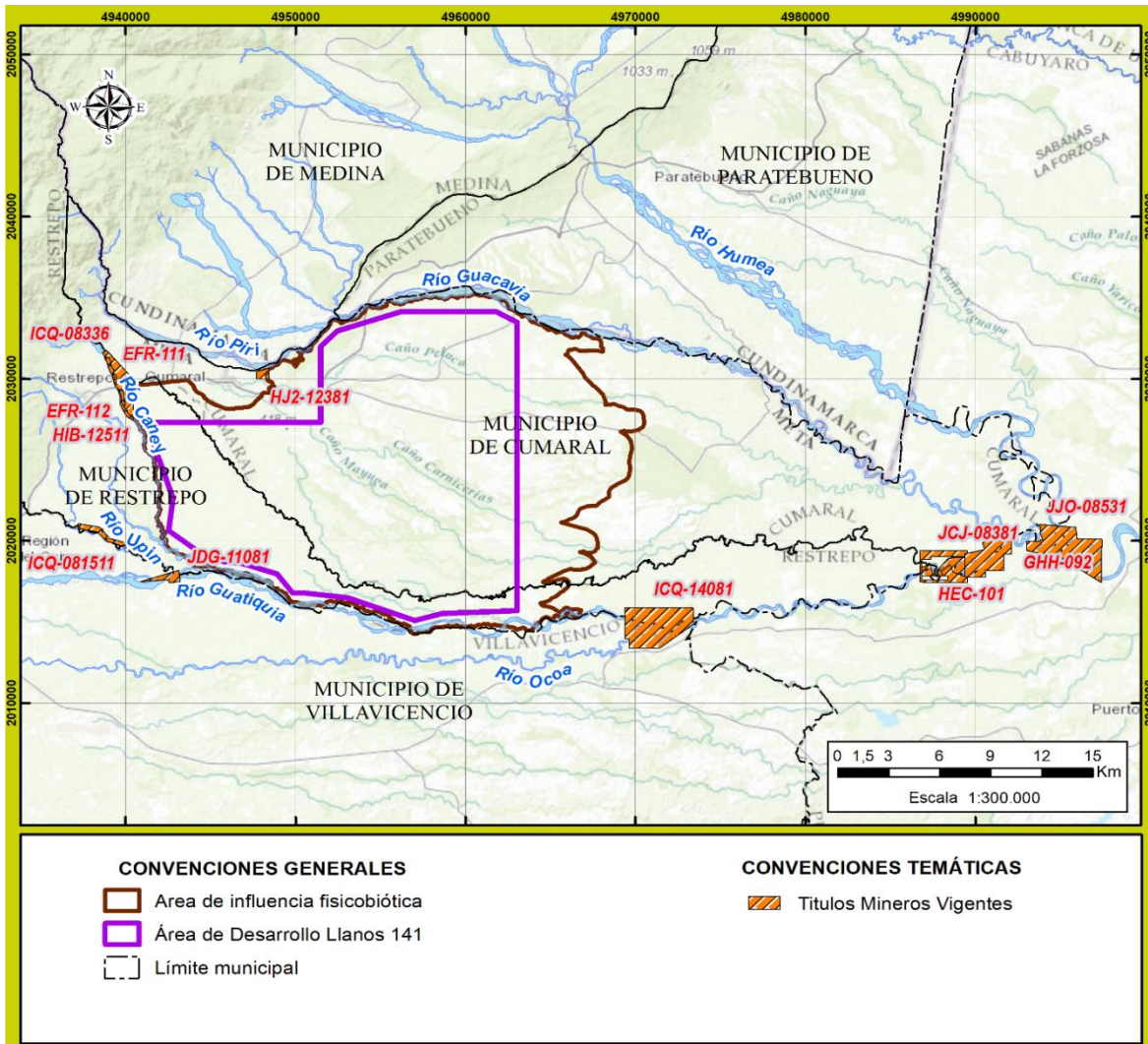
Figura 4.5-3 Ubicación fuentes de material de arrastre
